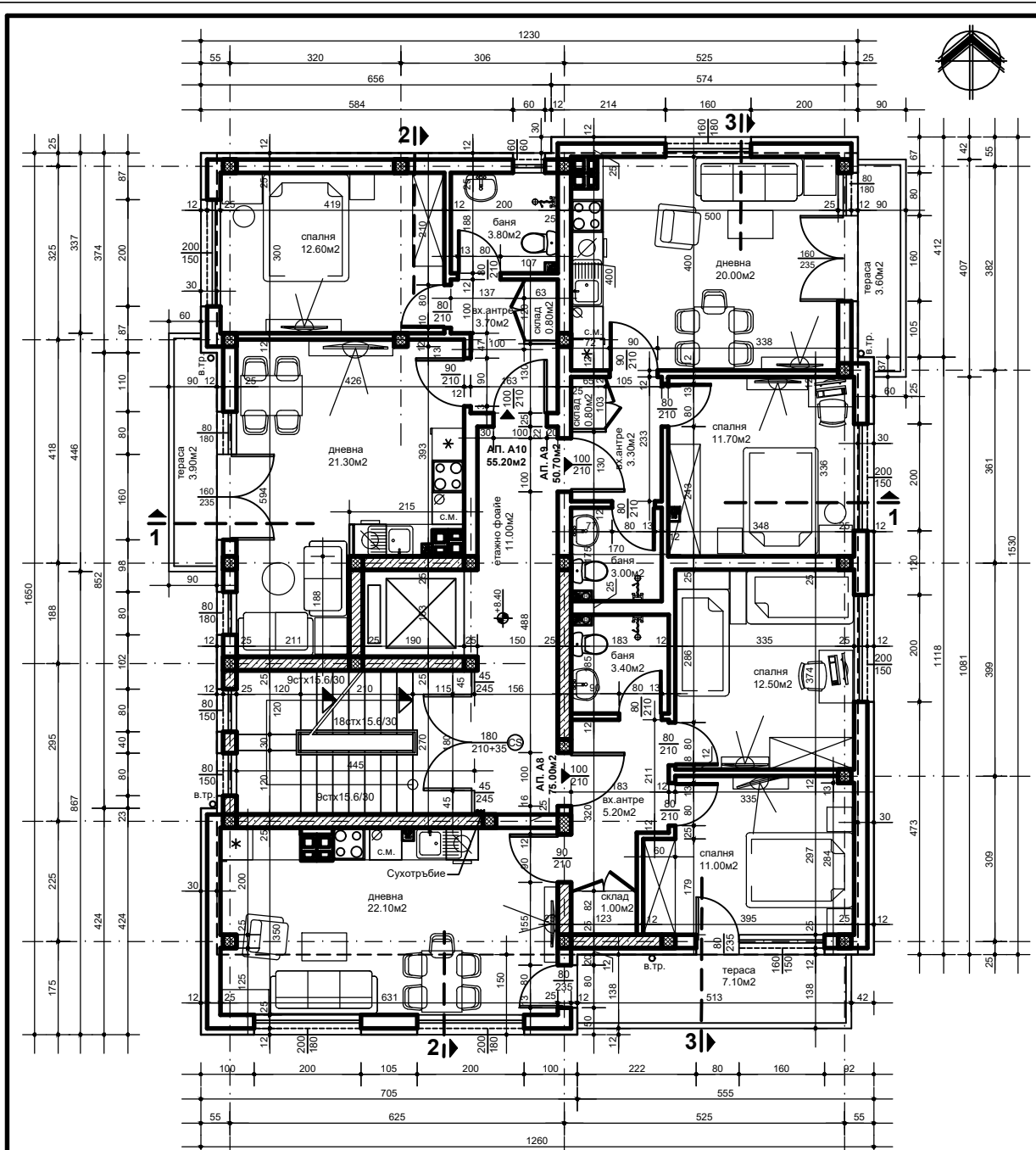
РАЗПРЕДЕЛЕНИЕ ЧЕТВЪРТИ ЕТАЖ - КОТА +8.40 - СГРАДА "А" М 1 : 50
