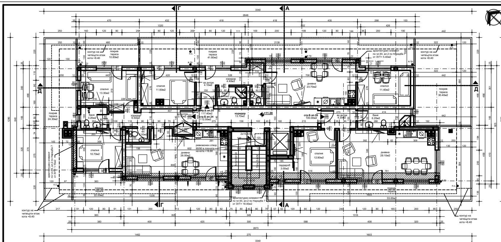
ЖИЛИЩНА СГРАДА Б - РАЗПРЕДЕЛЕНИЕ МАНСАРДЕН ЕТАЖ - КОТА +11.20 M 1 : 50
