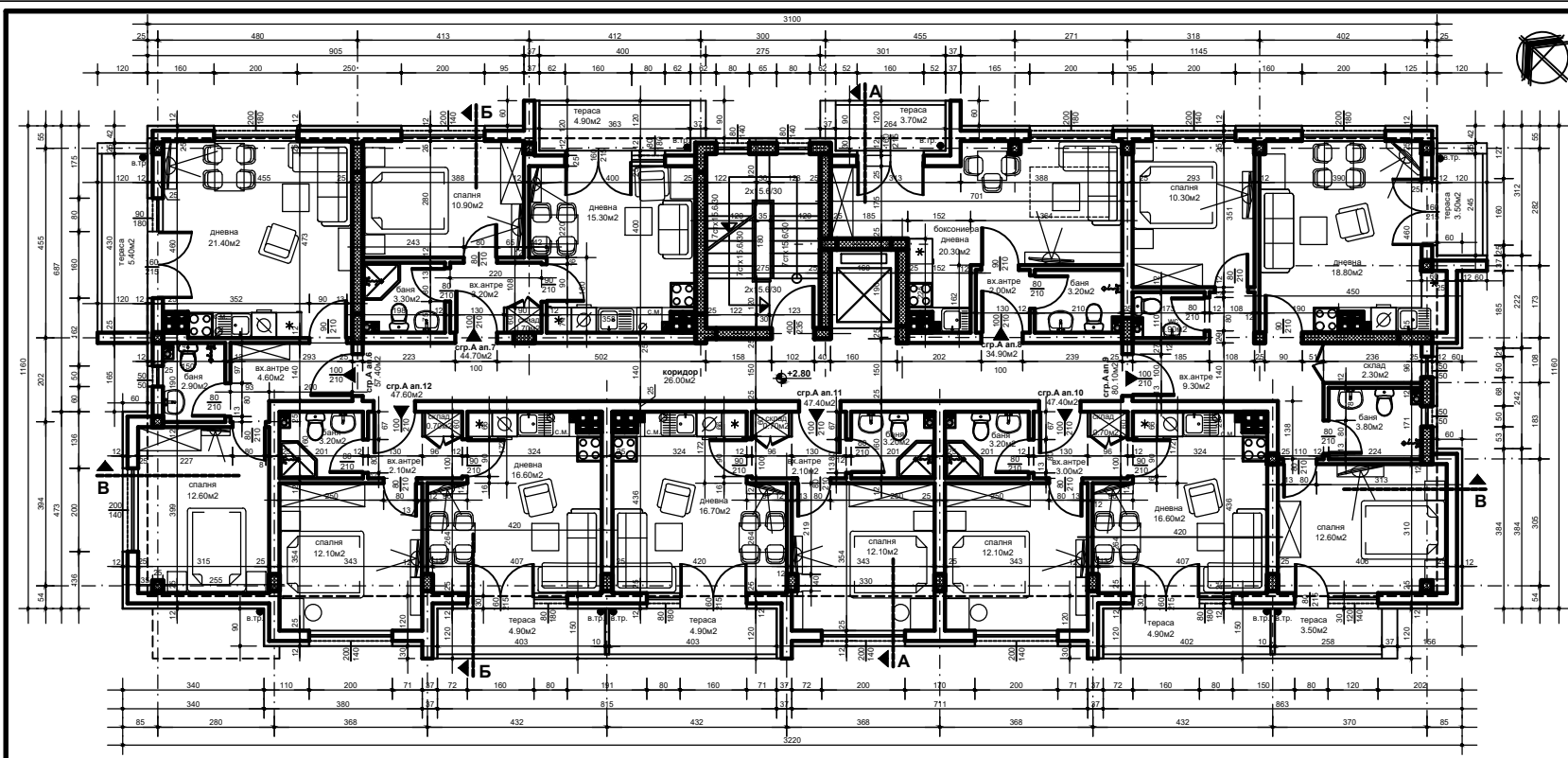
ЖИЛИЩНА СГРАДА А - РАЗПРЕДЕЛЕНИЕ ВТОРИ ЕТАЖ - КОТА +2.80 М 1 : 50
