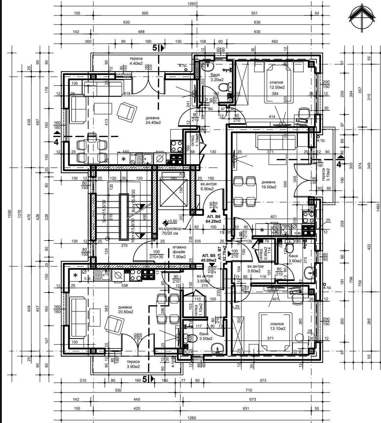
РАЗПРЕДЕЛЕНИЕ ТРЕТИ ЕТАЖ - КОТА +5.60 - СГРАДА "В"
