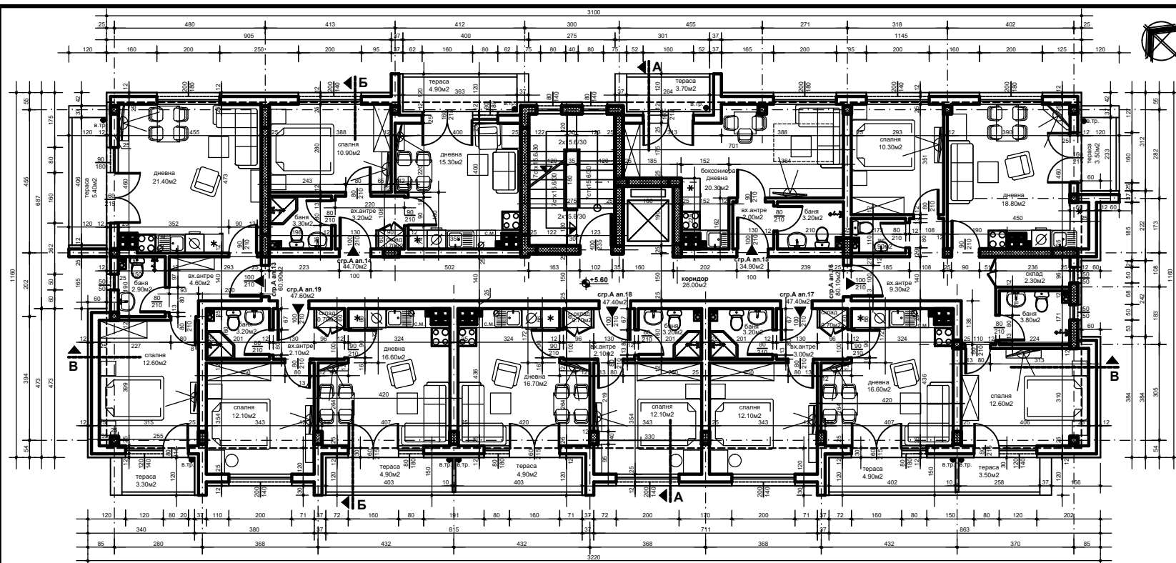
ЖИЛИЩНА СГРАДА А - РАЗПРЕДЕЛЕНИЕ ТРЕТИ ЕТАЖ - КОТА +5.60 М 1 : 50
