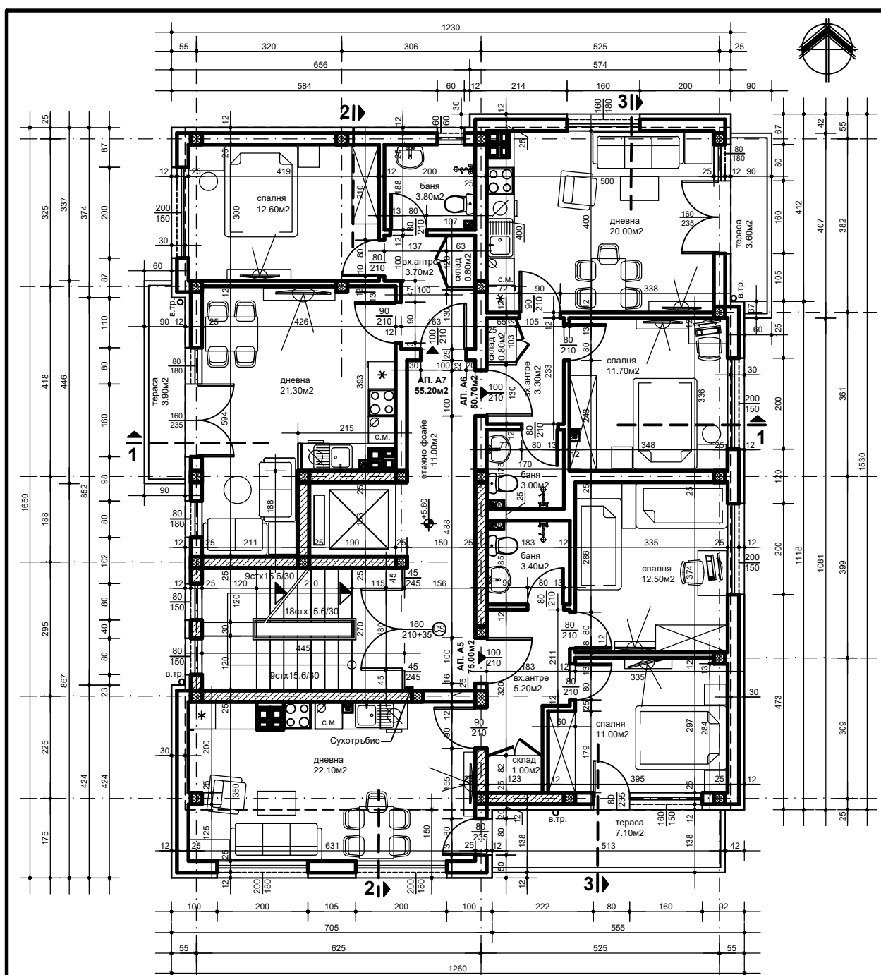
РАЗПРЕДЕЛЕНИЕ ТРЕТИ ЕТАЖ - КОТА +5.60 - СГРАДА "А" М 1 : 50
