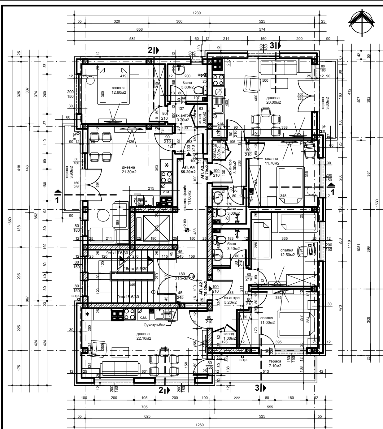
РАЗПРЕДЕЛЕНИЕ ВТОРИ ЕТАЖ - КОТА +2.80 - СГРАДА "А" М 1 : 50
