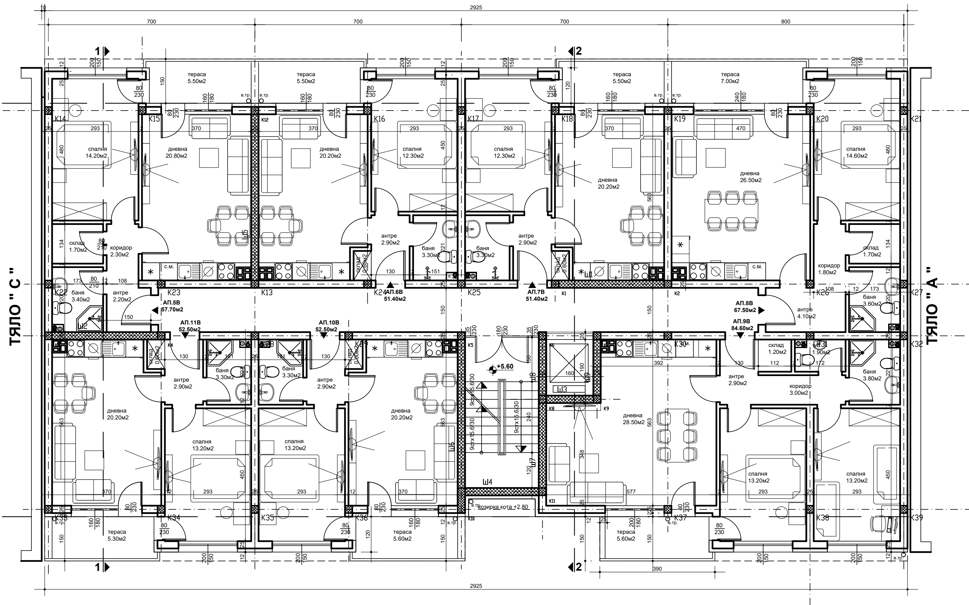
РАЗПРЕДЕЛЕНИЕ 2 этаж ТЯЛО " В " 3.П. 482.60м2 М 1:50
