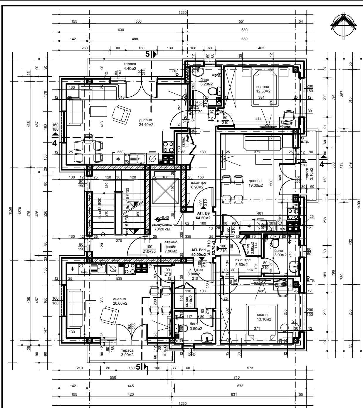
РАЗПРЕДЕЛЕНИЕ ЧЕТВЪРТИ ЕТАЖ - КОТА +8.40 - СГРАДА "В"
