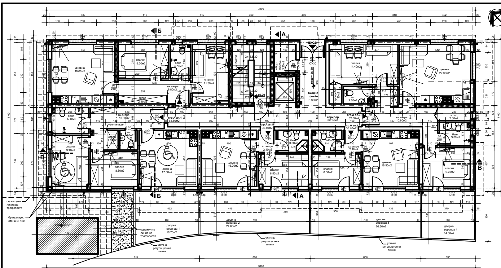
ЖИЛИЩНА СГРАДА А - РАЗПРЕДЕЛЕНИЕ ПЪРВИ ЕТАЖ - КОТА ±0.00 (ПАРТЕР) М 1 : 50
