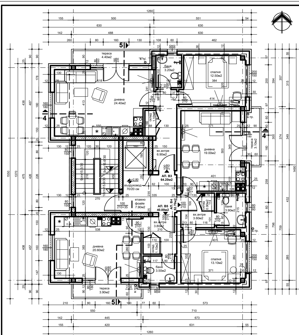
РАЗПРЕДЕЛЕНИЕ ВТОРИ ЕТАЖ - КОТА +2.80 - СГРАДА "В"
