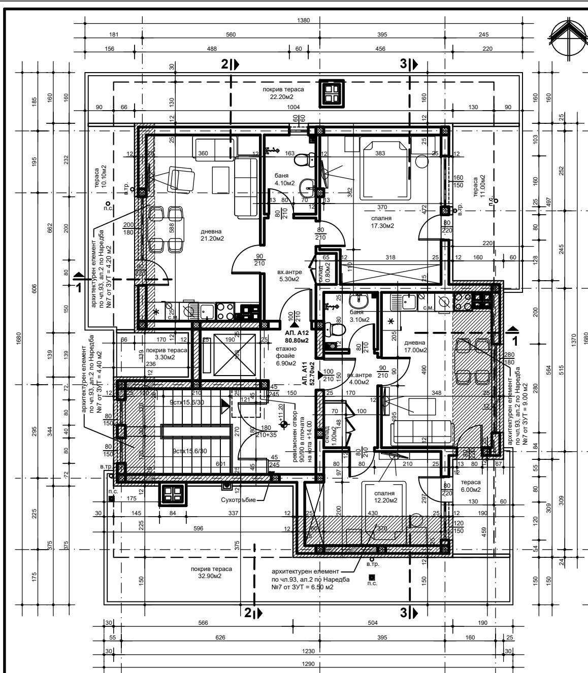
РАЗПРЕДЕЛЕНИЕ МАНСАРДЕН ЕТАЖ - КОТА +11.20 СГРАДА "А" М 1 : 50
