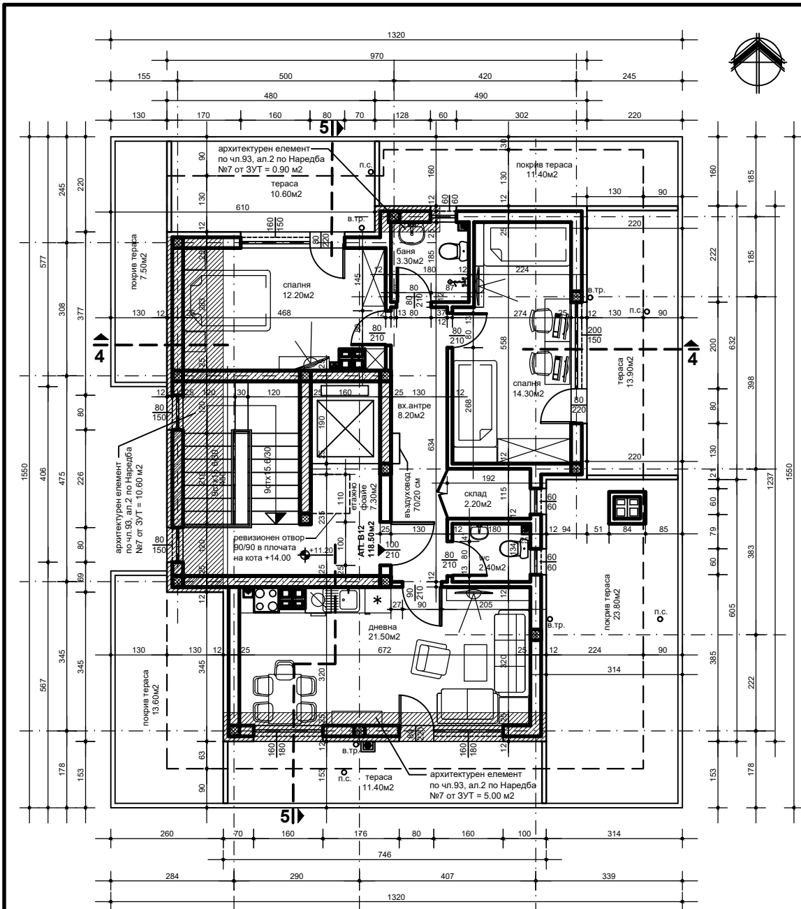
РАЗПРЕДЕЛЕНИЕ МАНСАРДЕН ЕТАЖ - КОТА +11.20 СГРАДА "В" М 1:50
