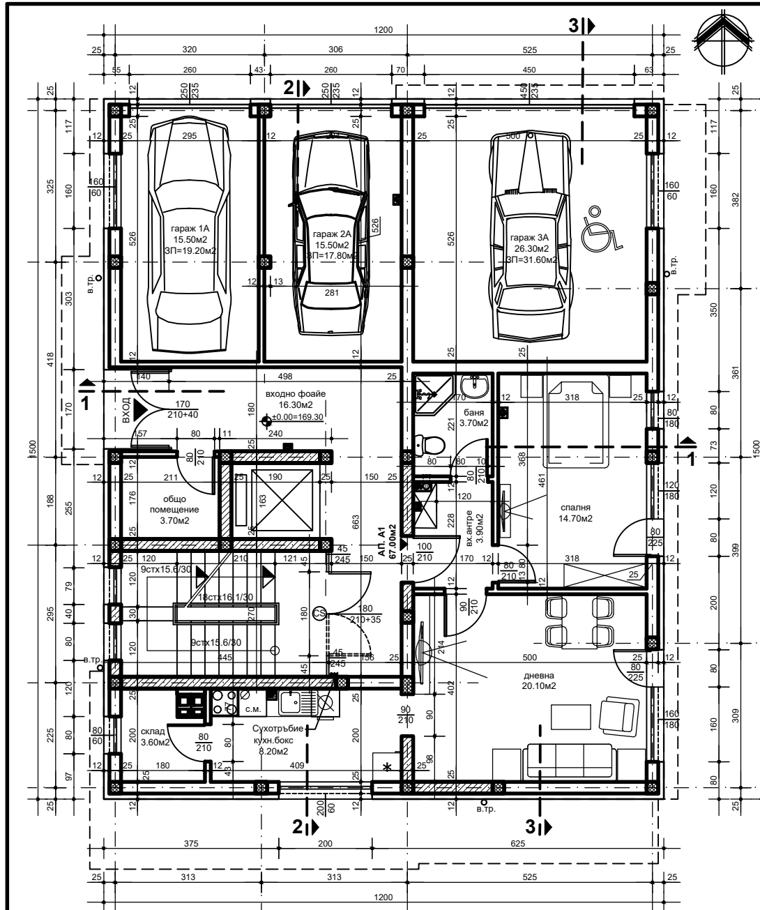
РАЗПРЕДЕЛЕНИЕ 1 ЕТАЖ - КОТА ±0.00 - СГРАДА "А" М 1 : 50
